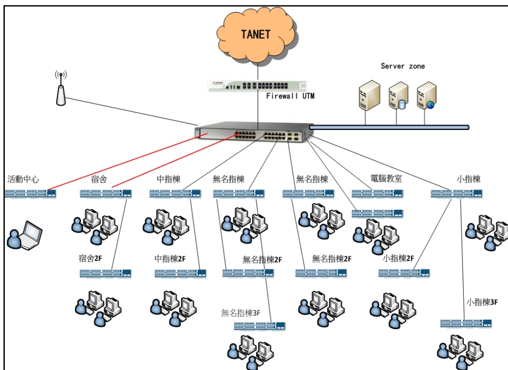
圖 1、國立南投特殊教育學校校園網路架構圖
